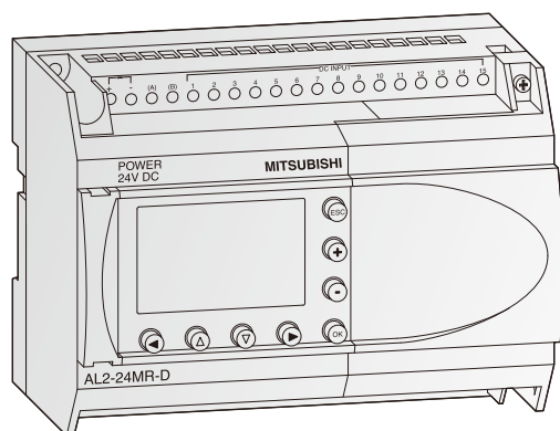
AL2-24MR-D
