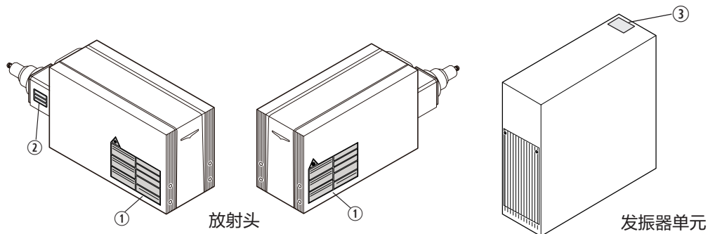
① 警告、说明、开口标签：LP-ZV200P/LP-ZV205P/LP-ZV206P
